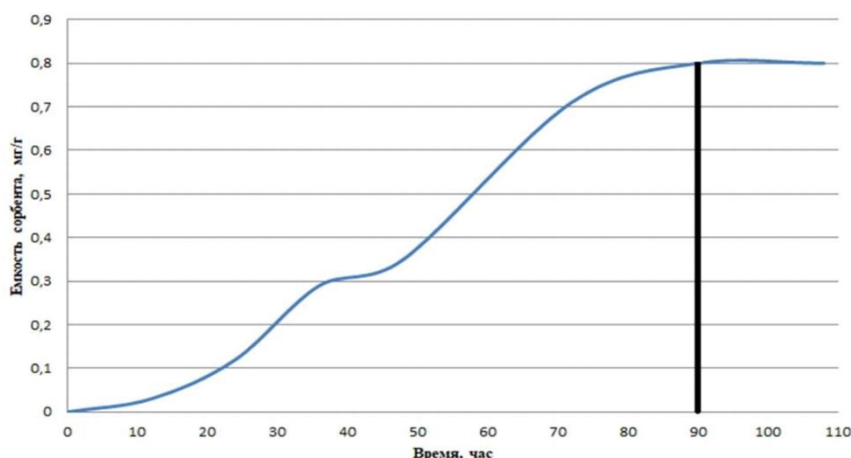
Рис. 2. Зависимость насыщения сорбента золотом от времени сорбции из оборотной воды с исходной концентрацией C_{исх.} = 0,035 мг/л
