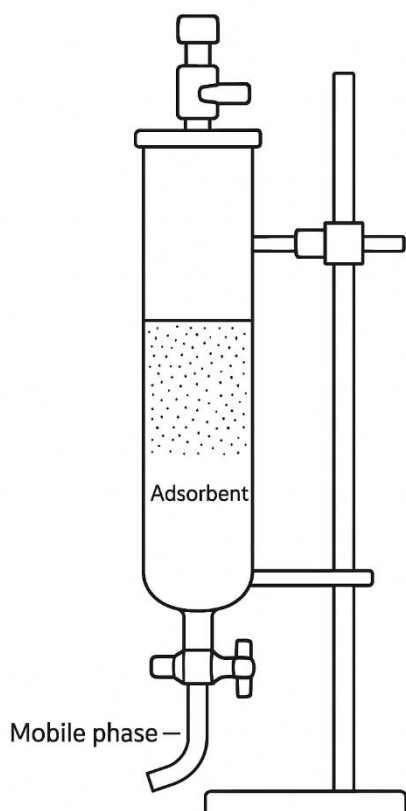
Рис. 1. Специальные лабораторные колонки для сорбции и хроматографии
