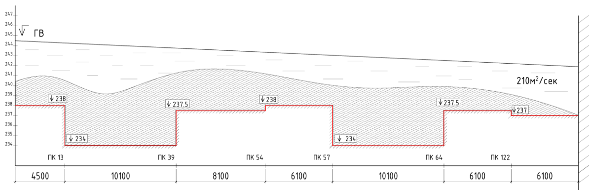
1-rasm. QMK ko'ndalang sxemasi tindirgich hovuzlar
