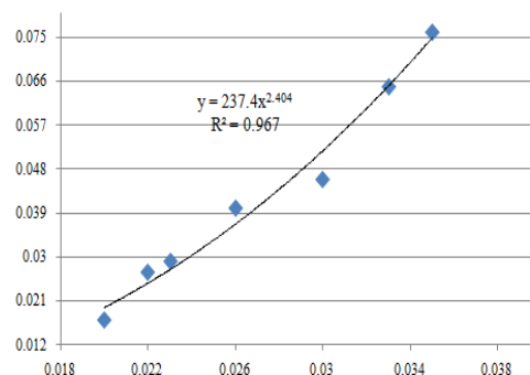
1-rasm. Tajribaviy gryadlarning balandligini hisobiy gryadlarning qiymatlari bilan taqqoslash
