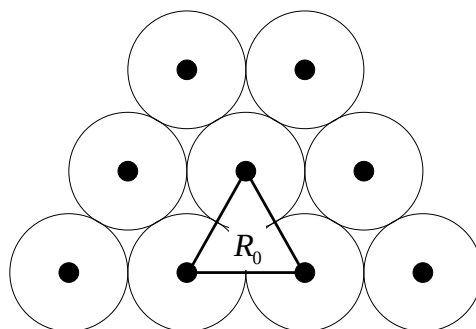
Рис.5. Покрывание плоскости окружностями с помощью треугольника
