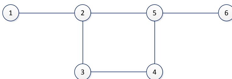
Рис.2. Пример графа
