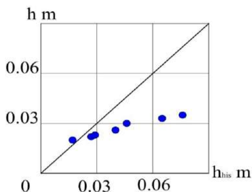
1-rasm. Tajribaviy gryadlarning balandligini hisobiy gryadlarning qiymatlari bilan taqqoslash
