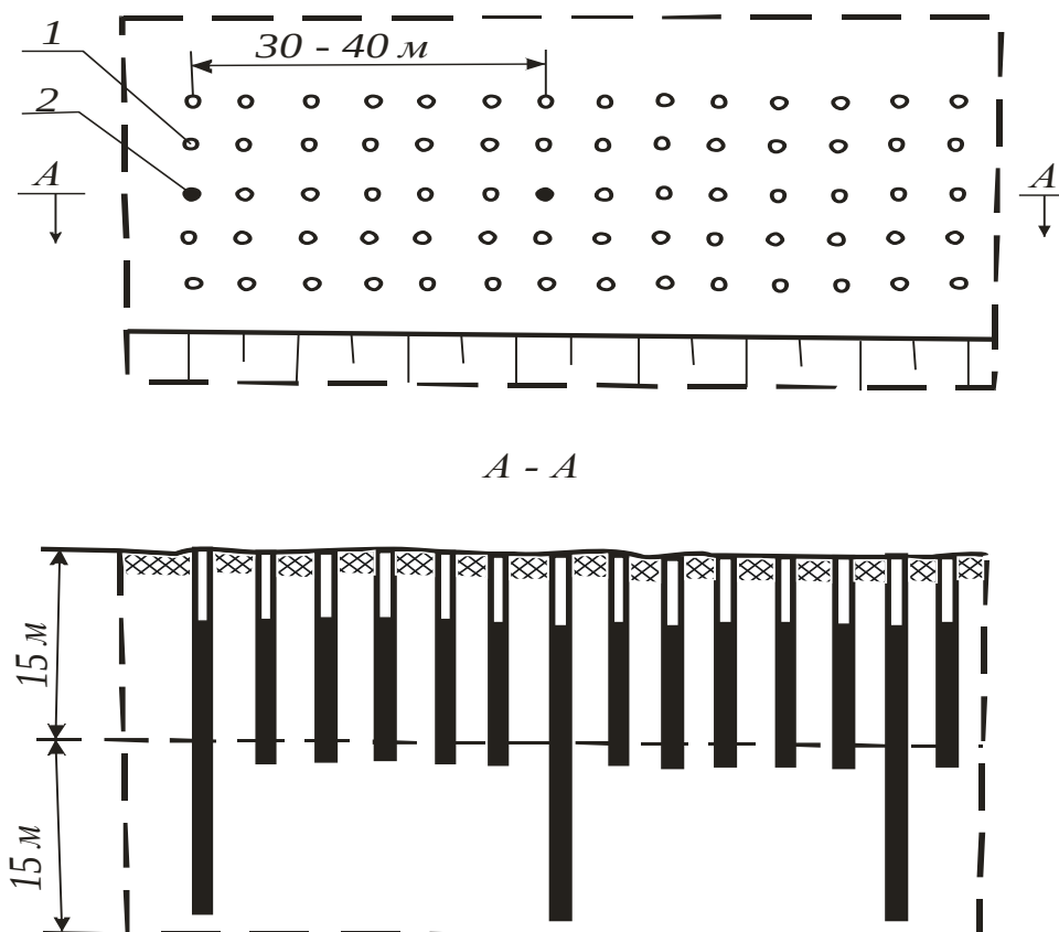
Рис. 2. Технология БВР с бурением части на глубину двух уступов
