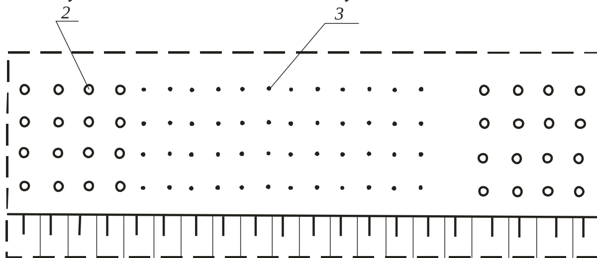
Рис. 3. Технология ведения буровзрывных работ путем предварительного осушения массива горных пород
