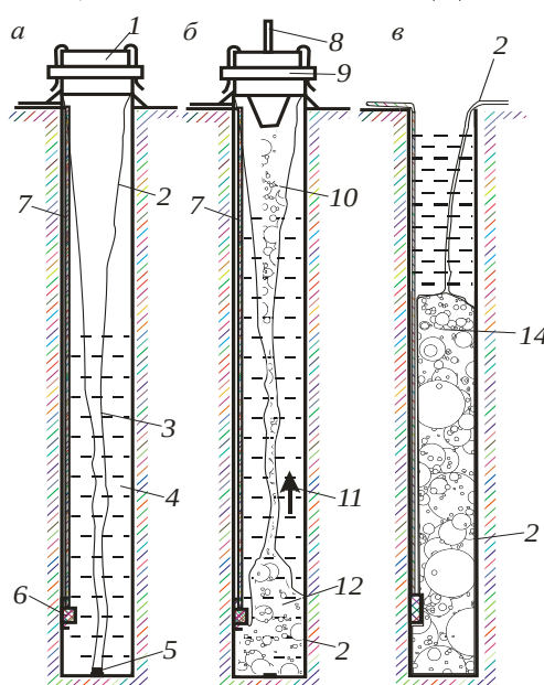
Рис. 1. Принципиальная схема формирования гидроизолированного заряда ВВ в обводненной скважине
