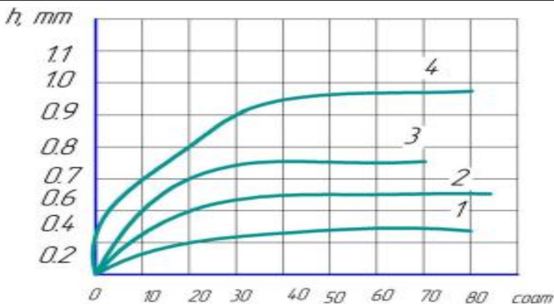
2-расм. Азотланган 38Х2МЮА маркали пўлатни қалинлиги ва температураси 0С 1-500; 2-525; 3-550; 4-600.
